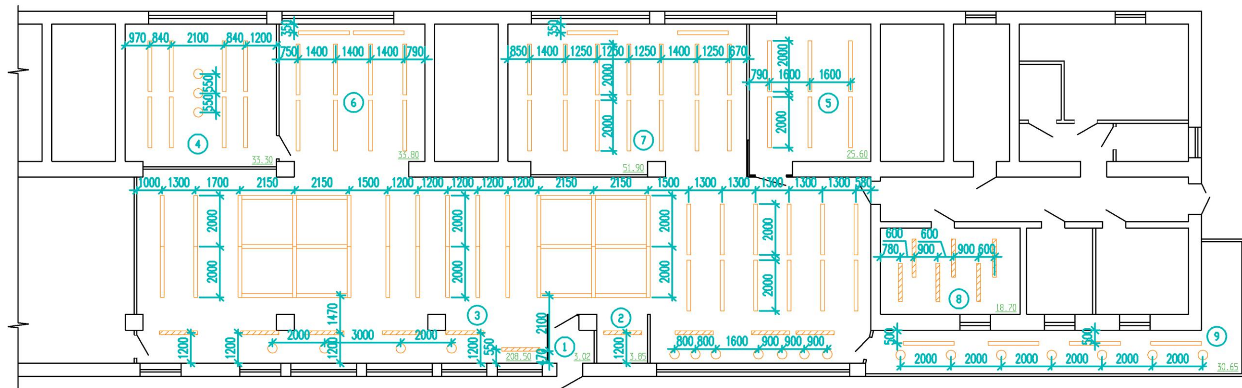
Экспликация осветительных приборов
