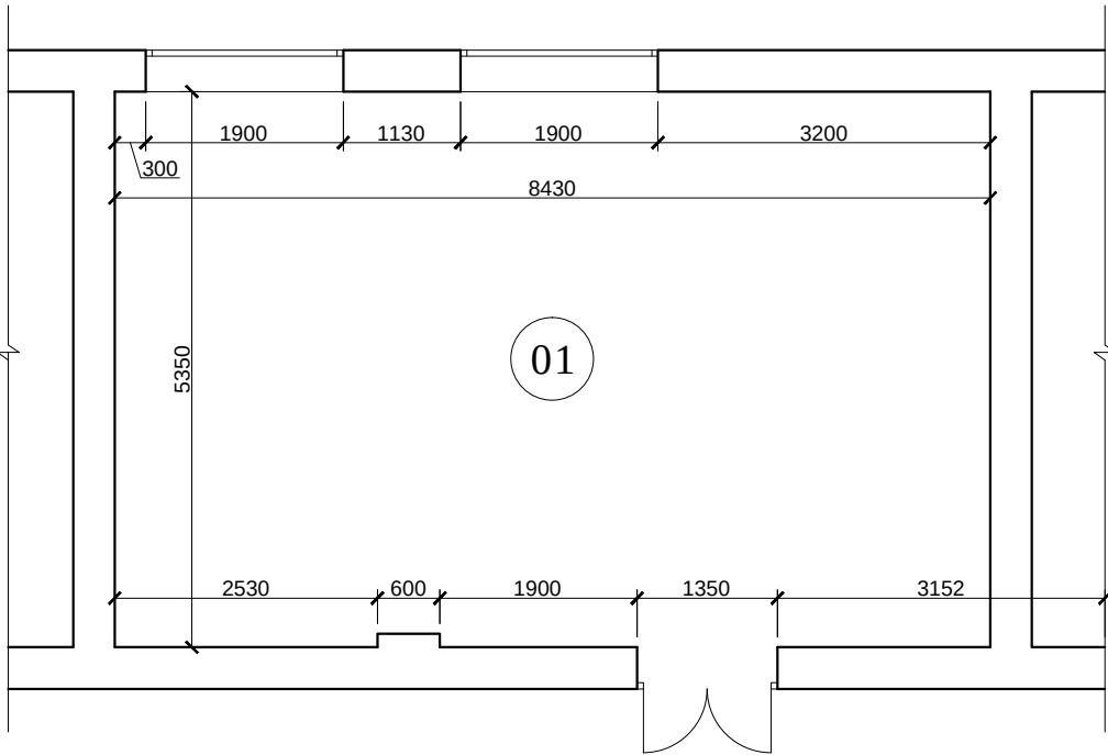
Фрагмент плана 1
