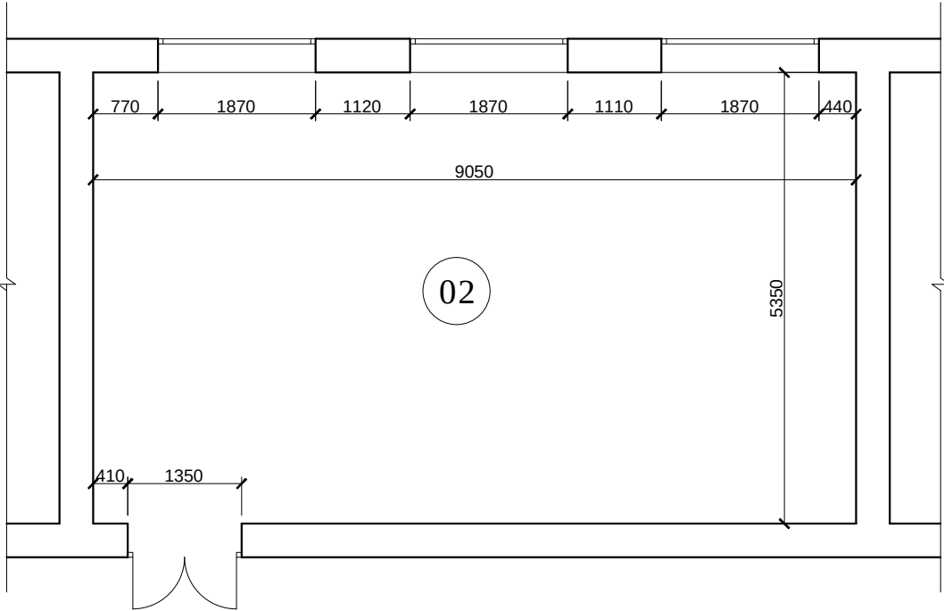
Фрагмент плана 2
