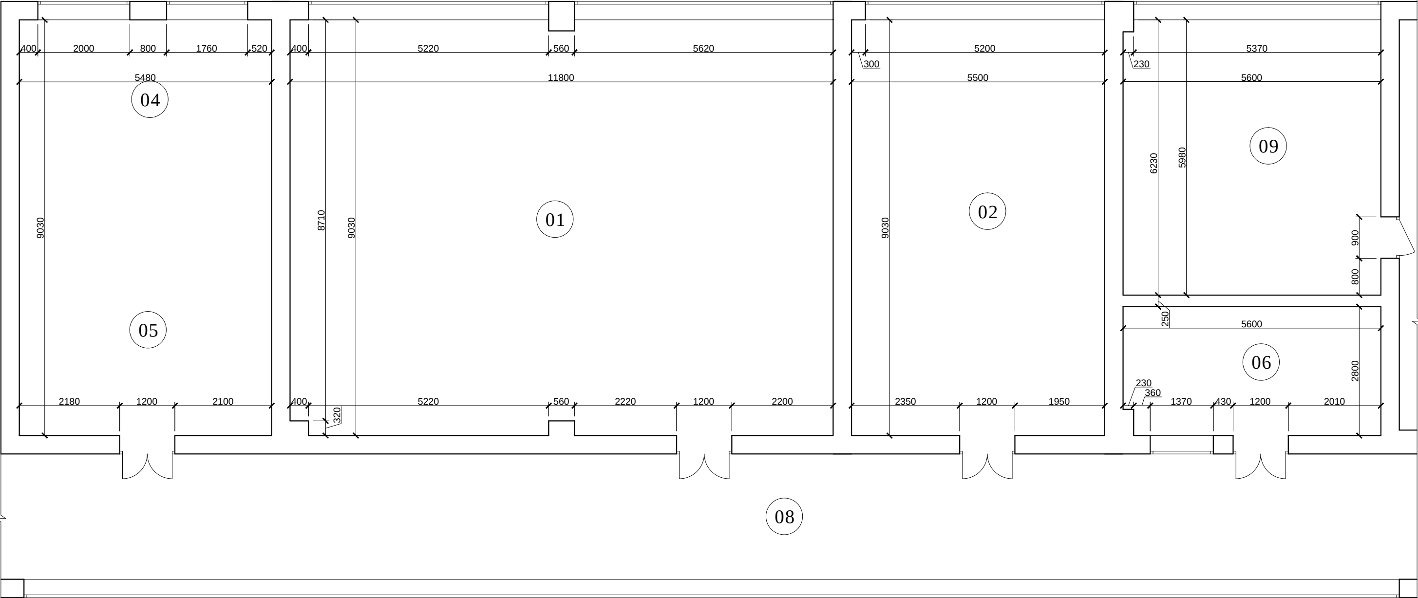
Экспликация помещений
