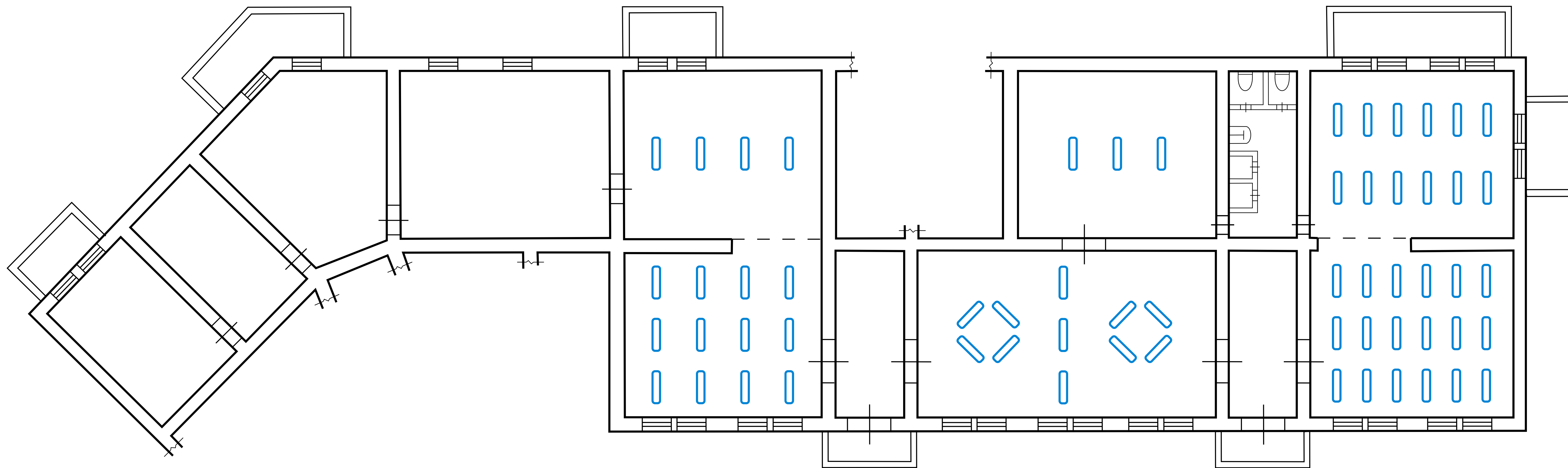
План расстановки светильников
