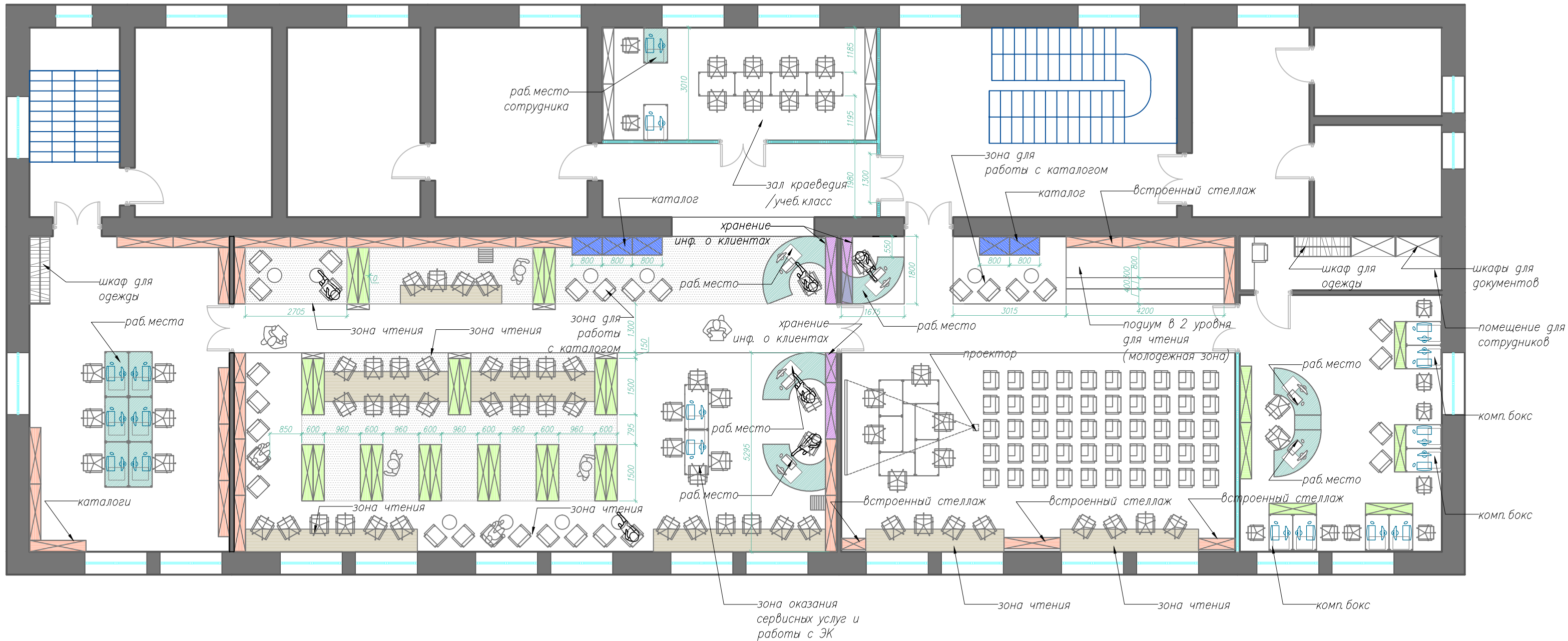
Планировка 2 этажа библиотеки
