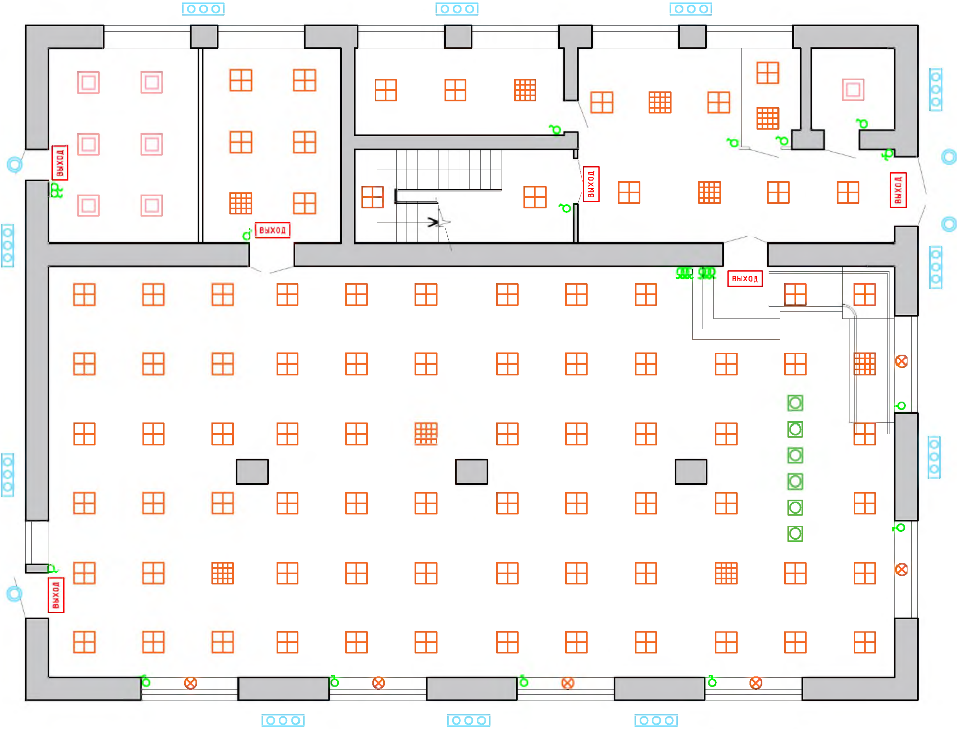
СПЕЦИФИКАЦИЯ СВЕТИЛЬНИКОВ И ПРИБОРОВ
