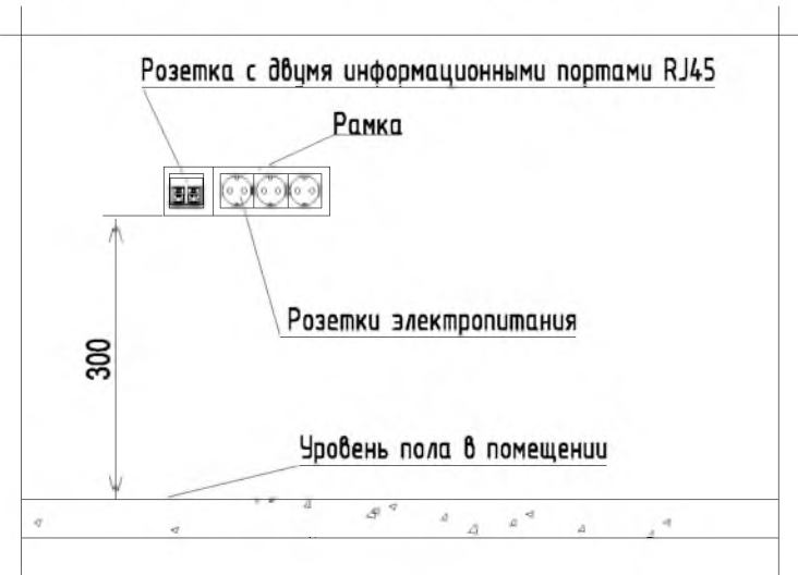
УСТАНОВКА ЭЛЕКТРОРОЗЕТОК НА СТЕНЕ
