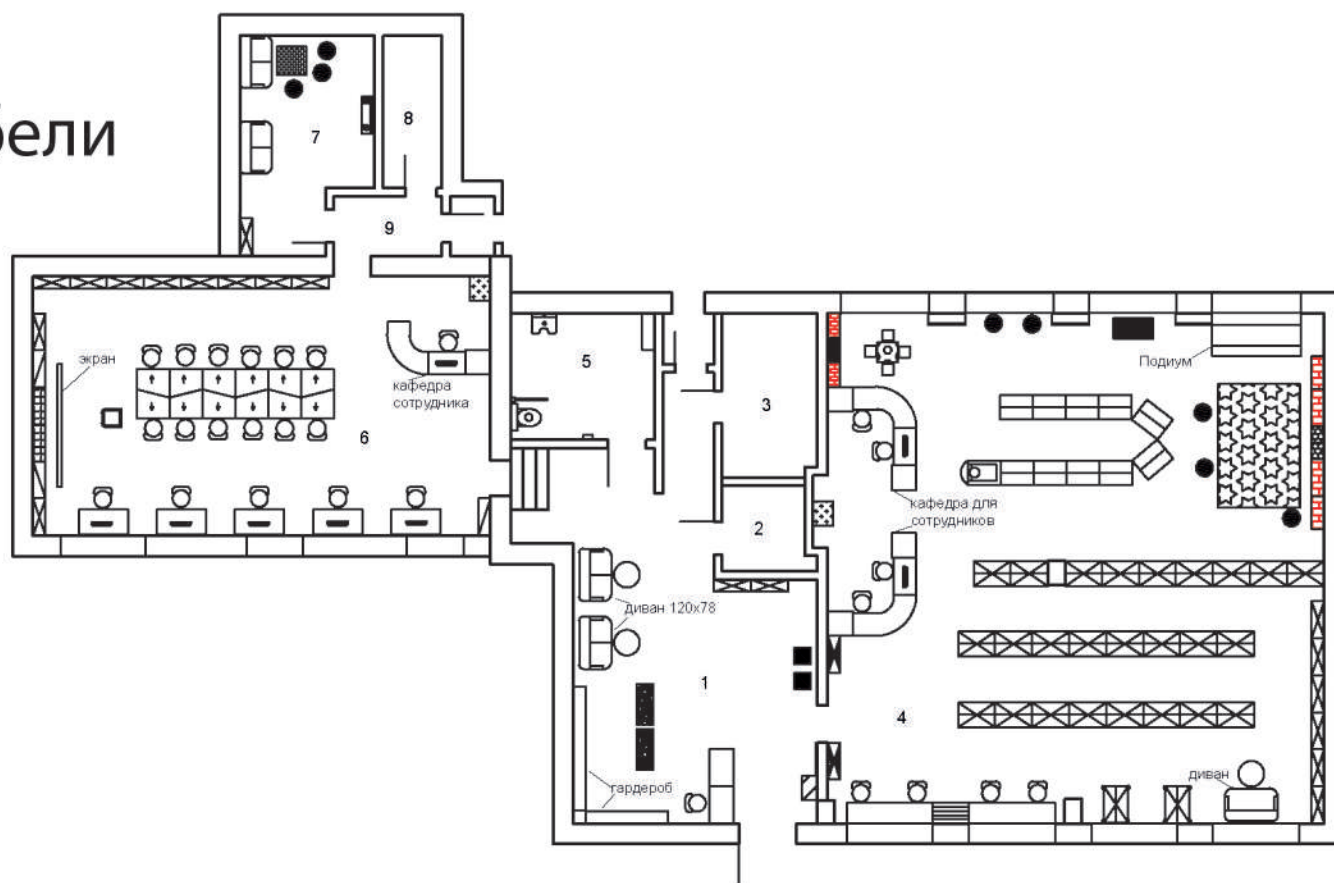
Экспликация помещений
