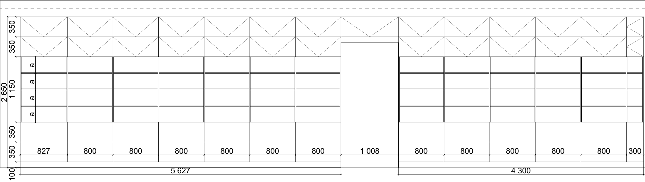
Фасад 4
