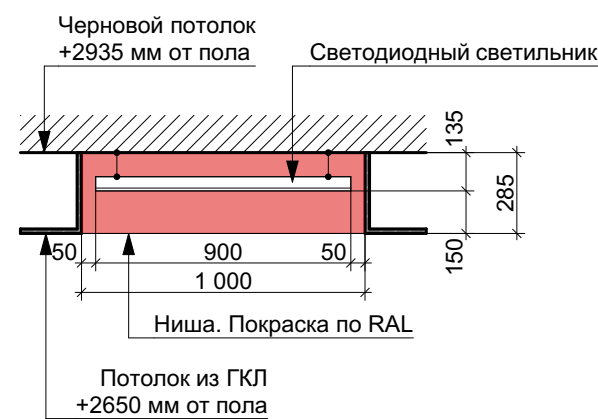
Разрез 1-1
