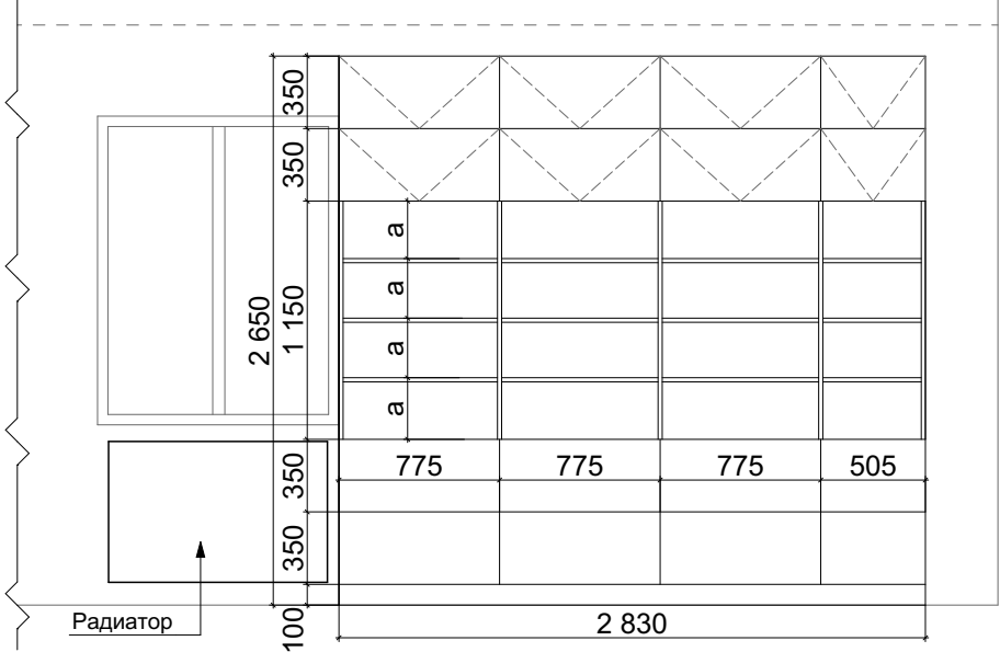
Фасад 2
