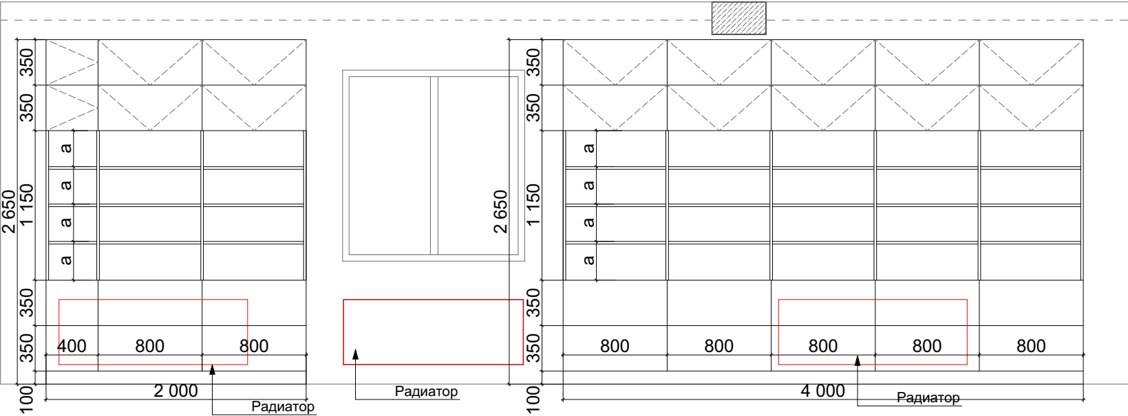
Фасад 3
