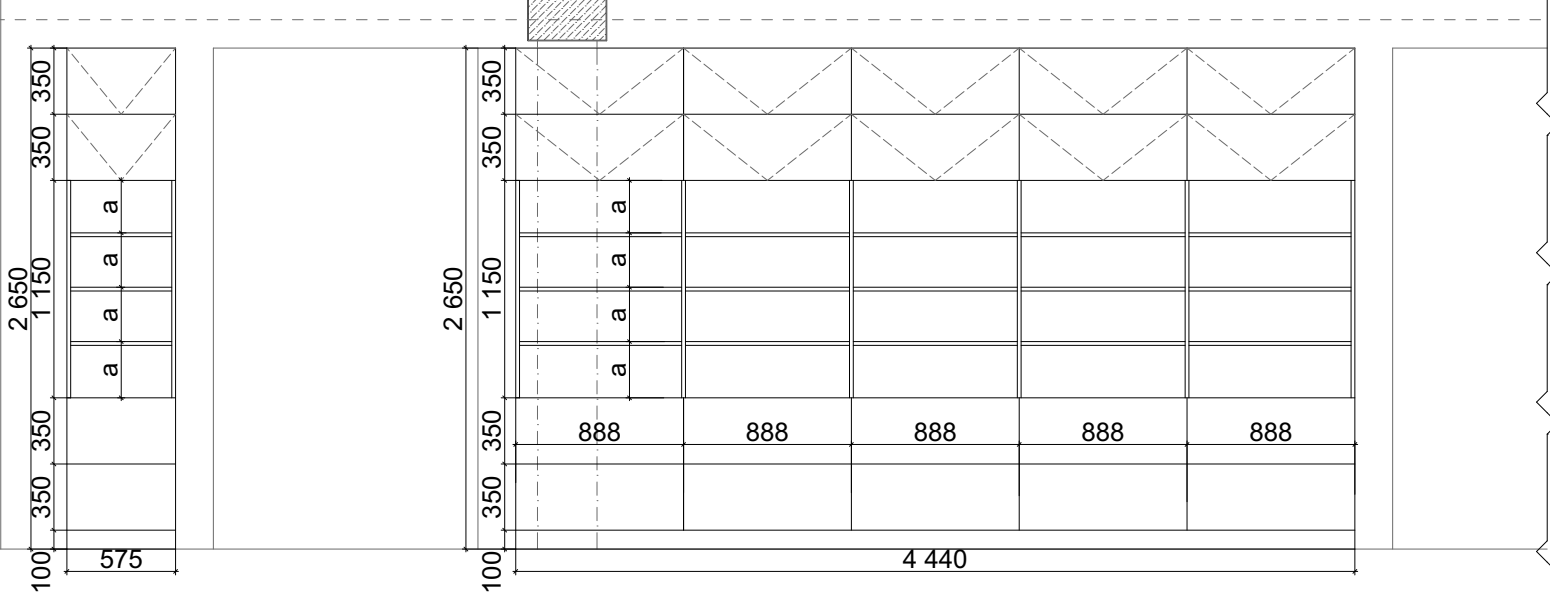
Фасад 4
