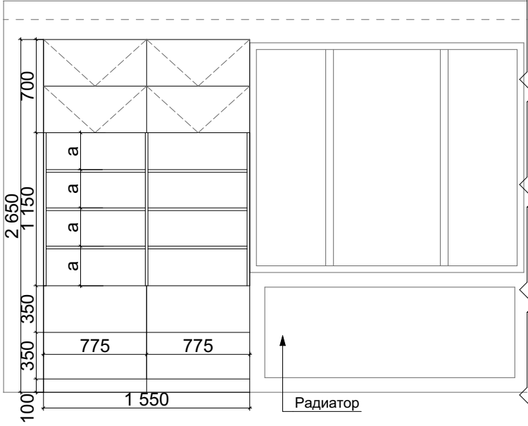
Фасад 2
