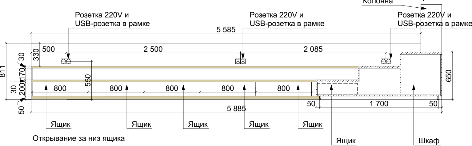
Разрез 2-2
