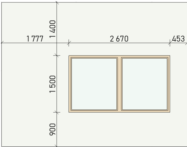
СТЕНА Г-А
