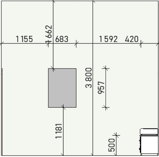
СТЕНА В-Г
