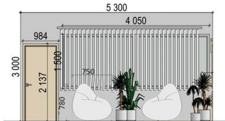
Стена В-Г
