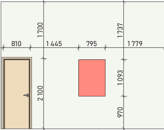
СТЕНА В-Г
