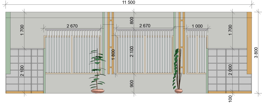
Стена Д-Е 11 500
