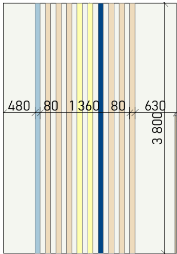
СТЕНА В-Г
