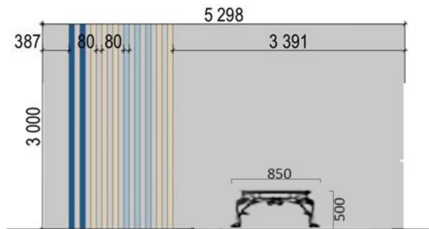
Стена В-Г
