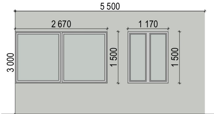
Стена Г-А
