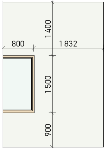
СТЕНА В-Г
