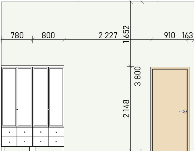
СТЕНА В-Г
