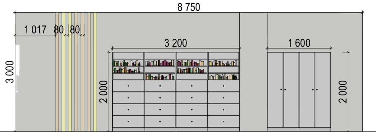
Стена В-Г
