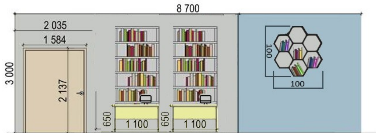
Стена В-Г
