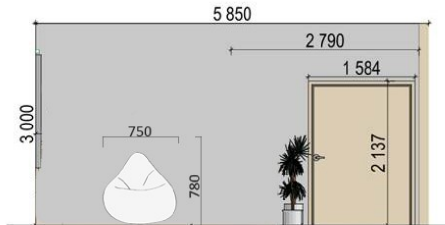
Стена Г-А
