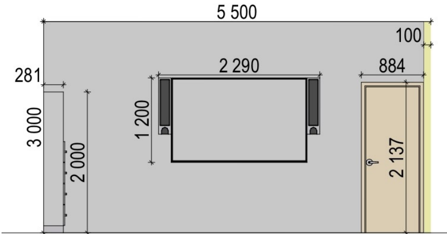
Стена Г-А
