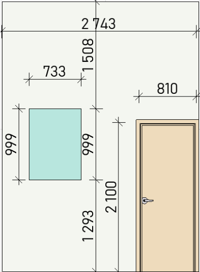
СТЕНА В-Г
