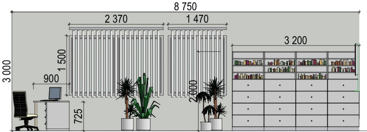
Стена В-Г
