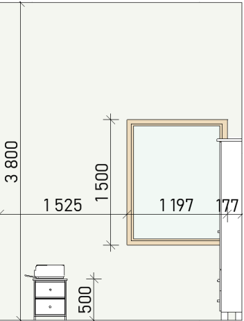
СТЕНА Г-А
