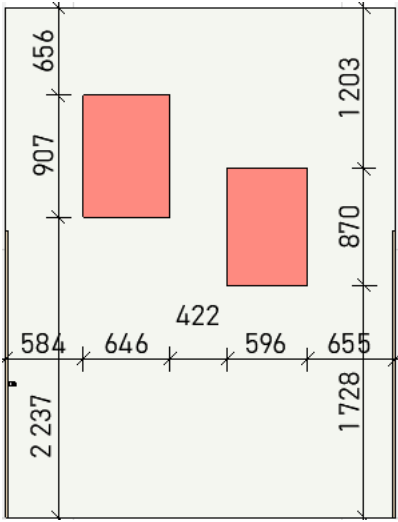
СТЕНА Г-А
