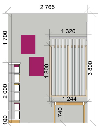
Стена Ж-3
