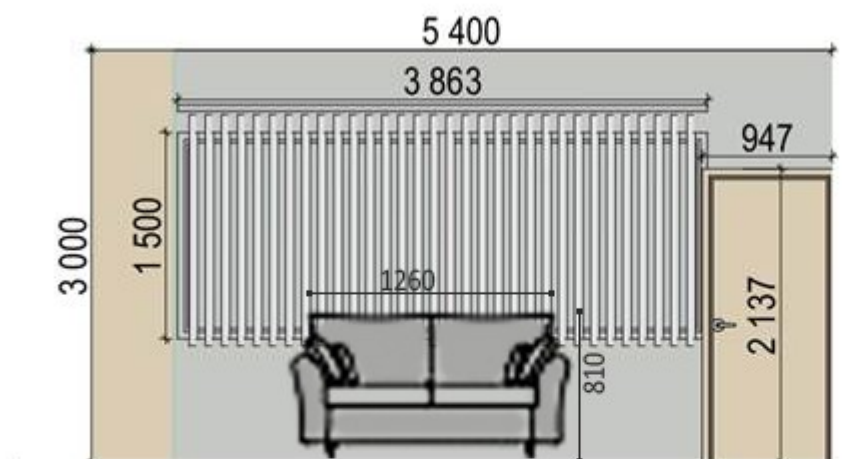
Стена Б-В
