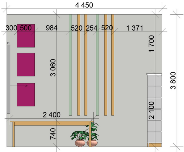
Стена Б-Ж
