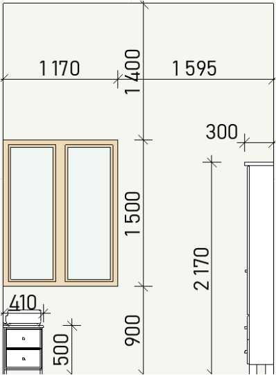
СТЕНА Г-А
