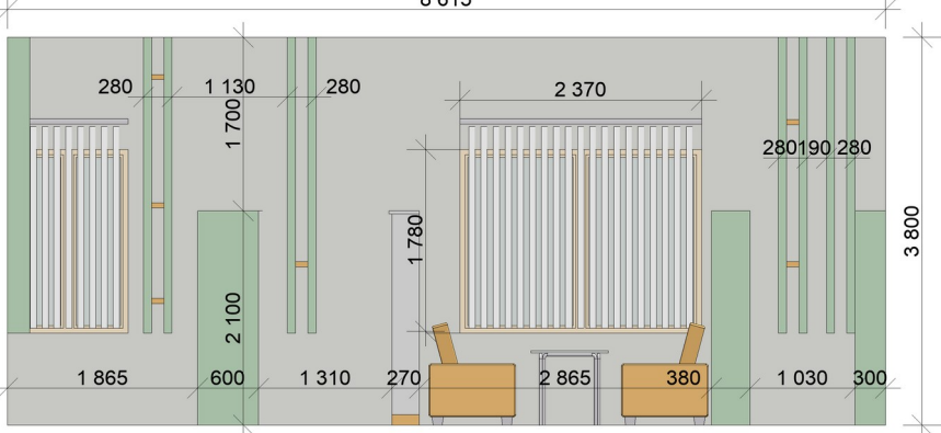
Стена Г-Д 8 615
