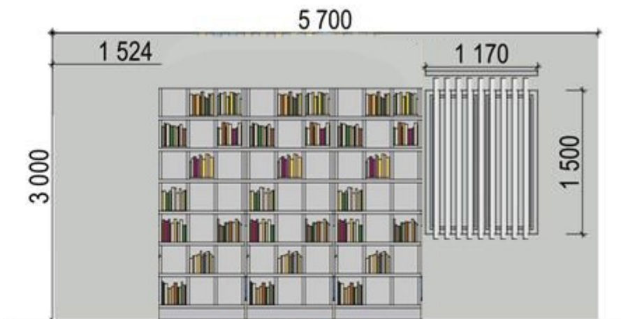
Стена Д-Е
