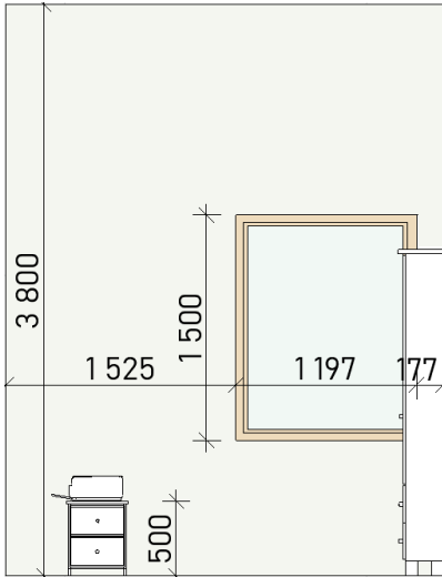
СТЕНА Г-А
