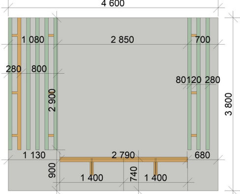
Стена В-Г 4 600
