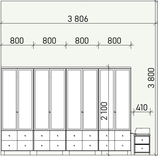
СТЕНА Г-А
