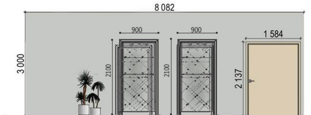
Стена В-А
