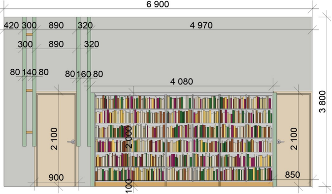
Стена А-Б 6 900
