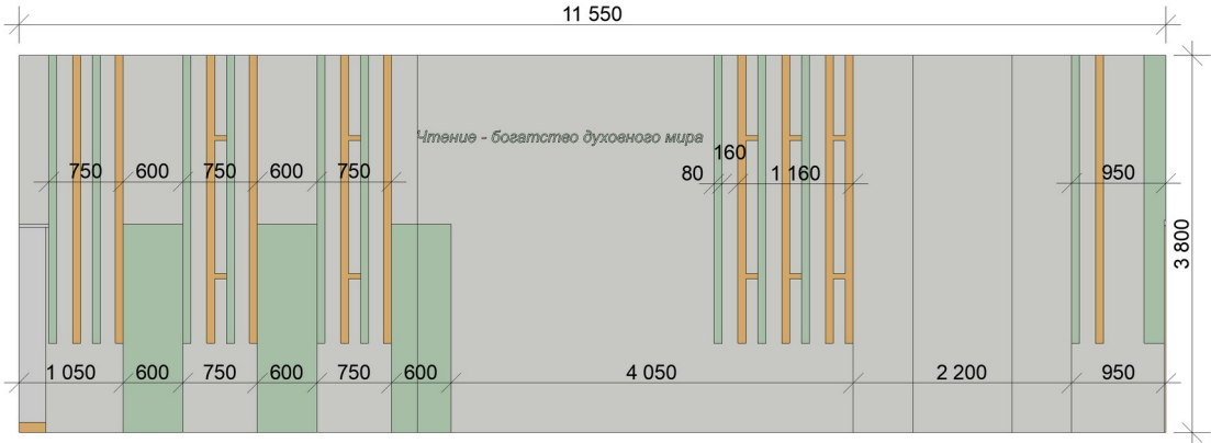
Стена Е-А 11 550
