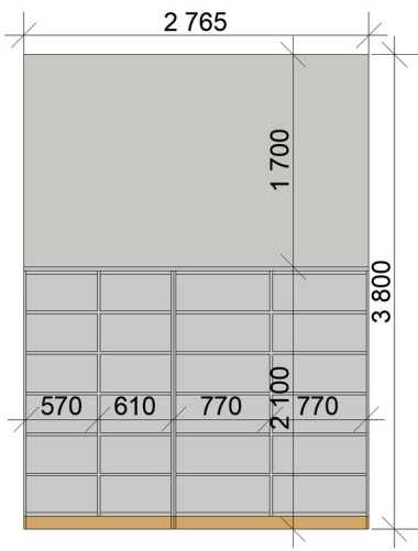
Стена Ж-3
