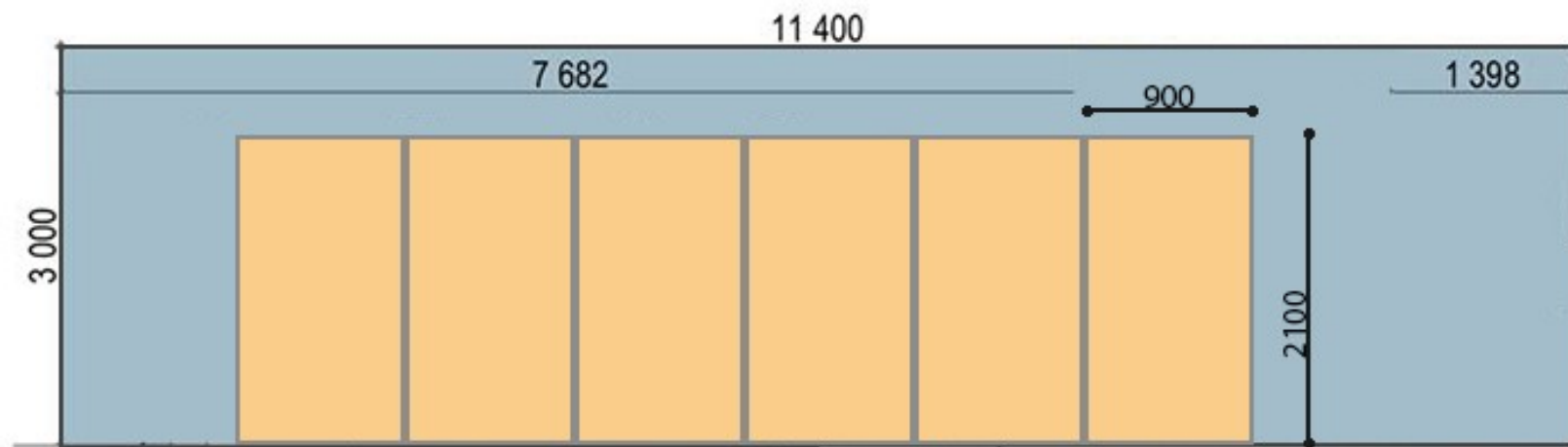
Стена В-Г
