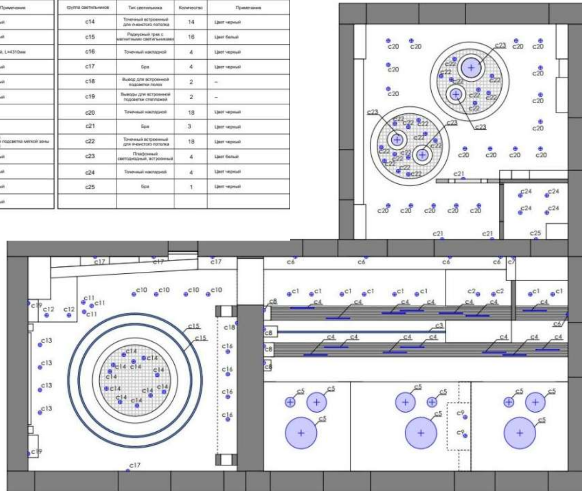
Ведомость светильников
