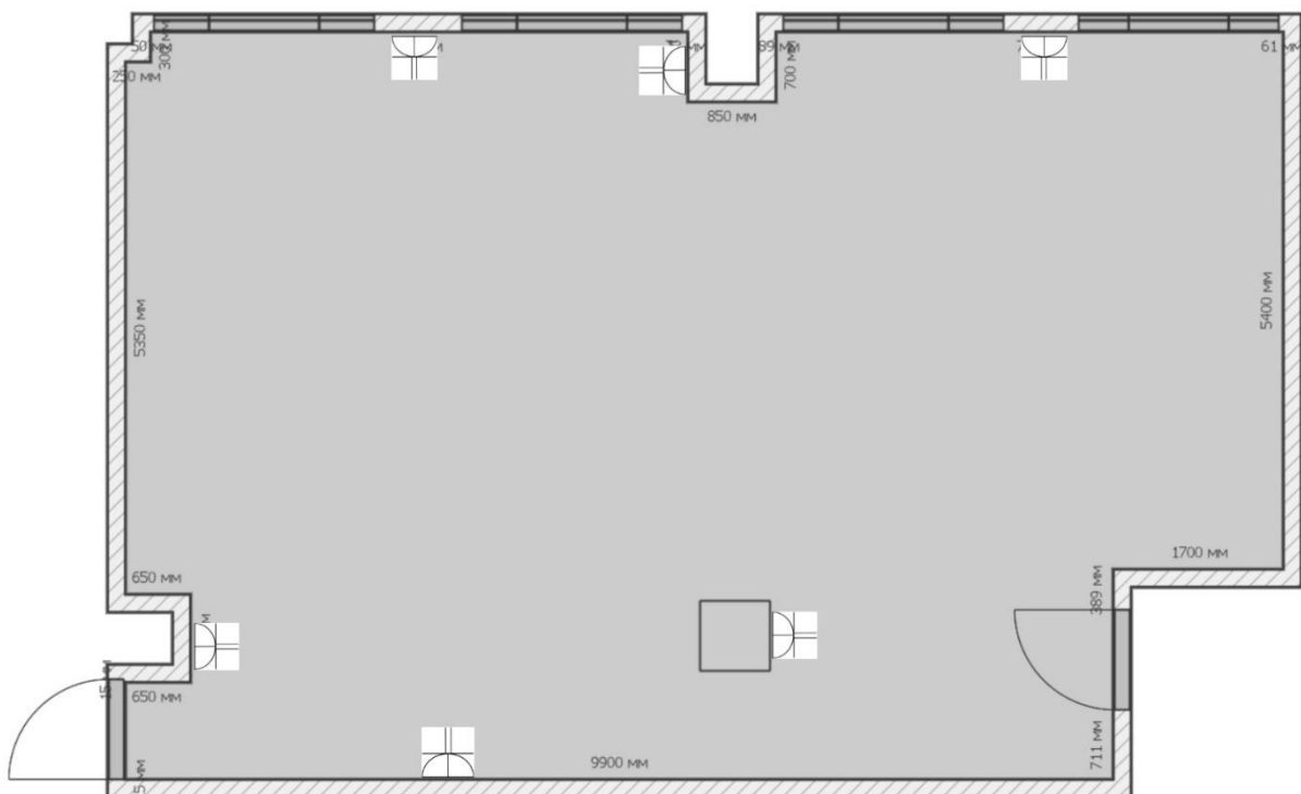
План расположения розеток
