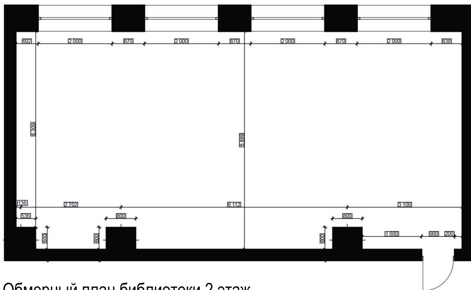
Обмерный план библиотеки 2 этаж
