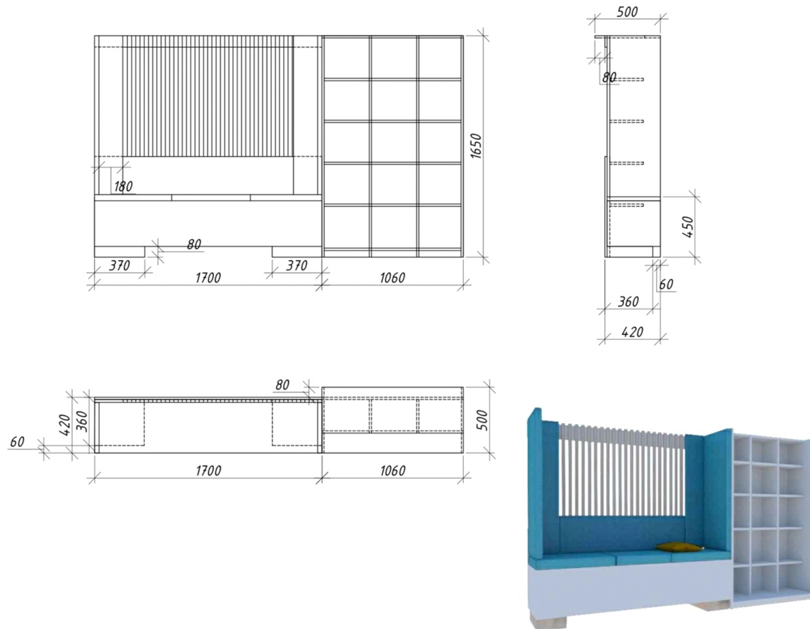
СТЕЛЛАЖ С РАБОЧИМ МЕСТОМ ДЛЯ ЧИТАЛЬНОГО ЗАЛА
