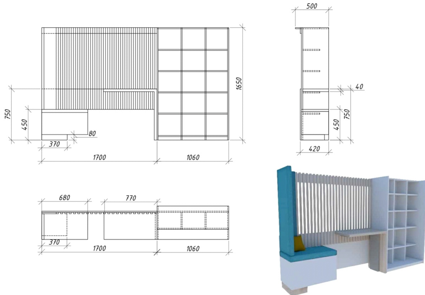
СТЕЛЛАЖ С РАБОЧИМ МЕСТОМ ДЛЯ ЧИТАЛЬНОГО ЗАЛА
