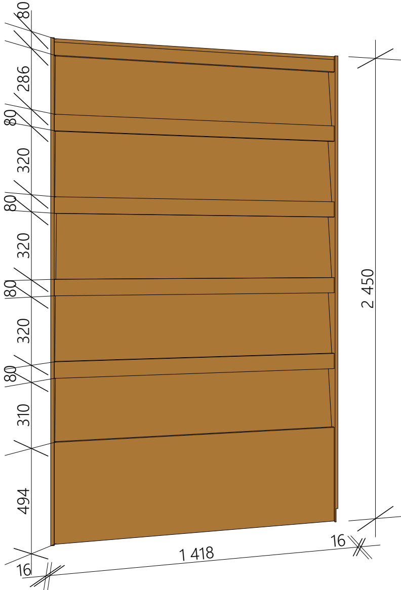
Шкаф 19 сторона 1
