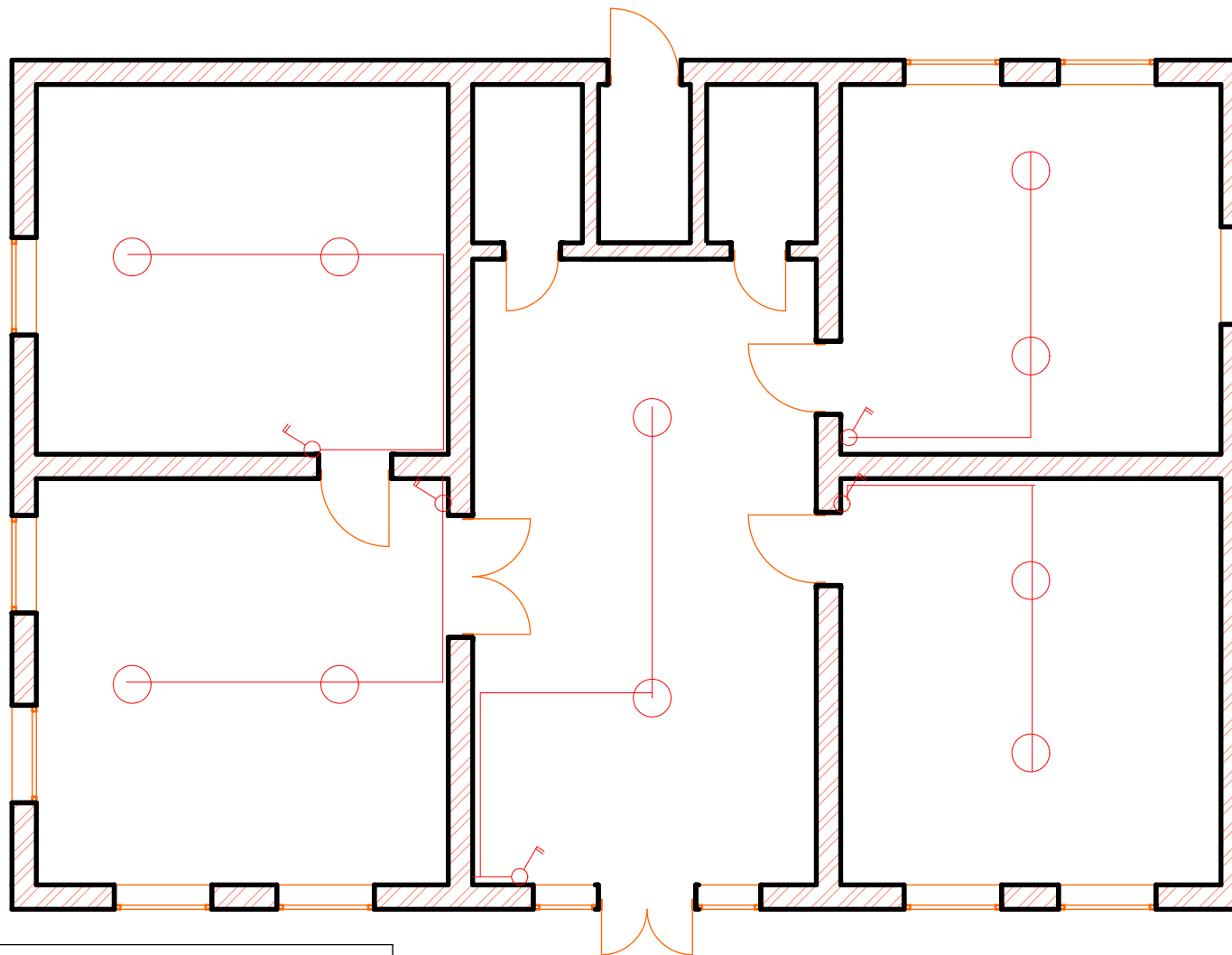
План освещения
