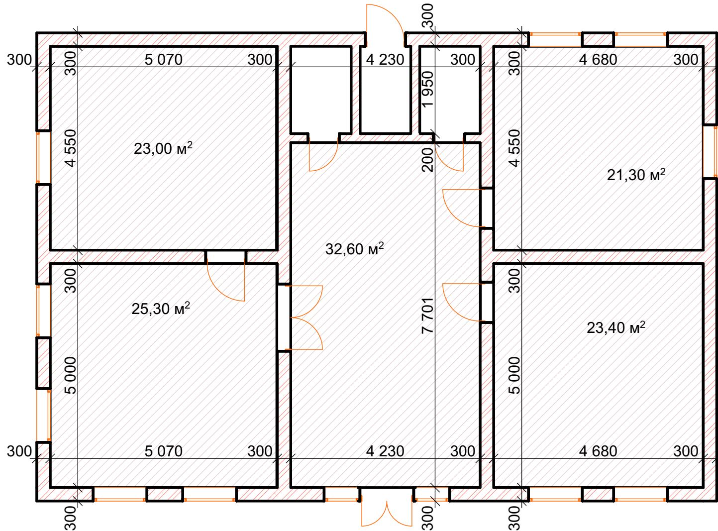
План обмерочный
