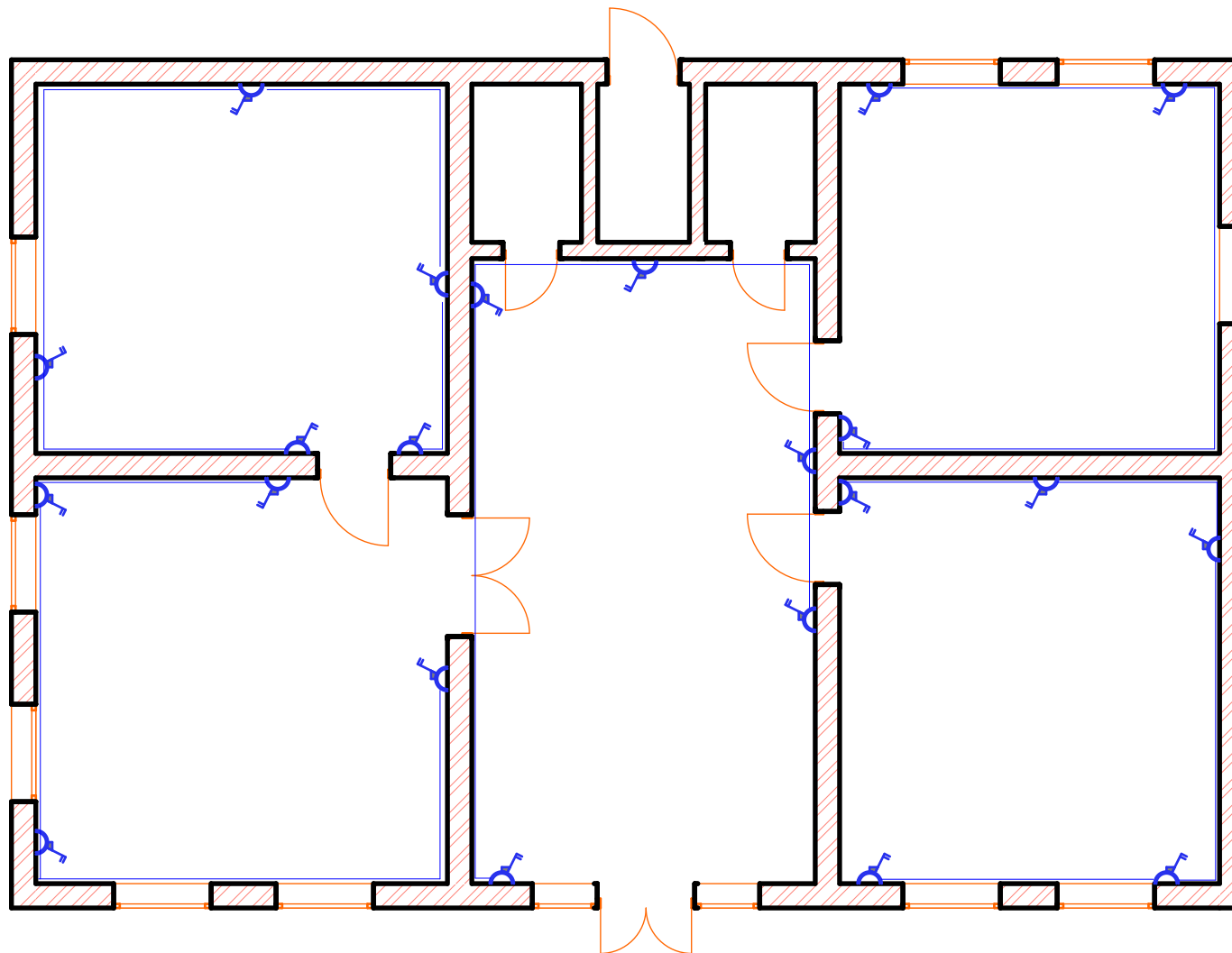
План розеток
