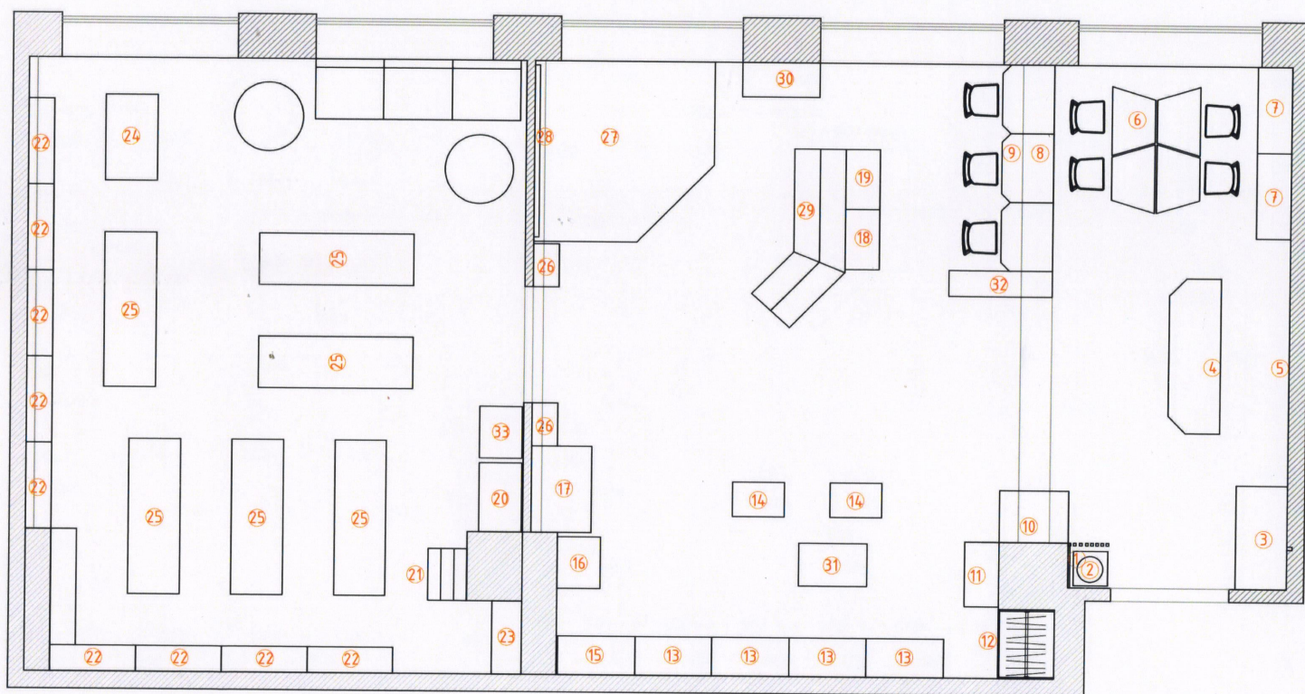
Планировочное решение
