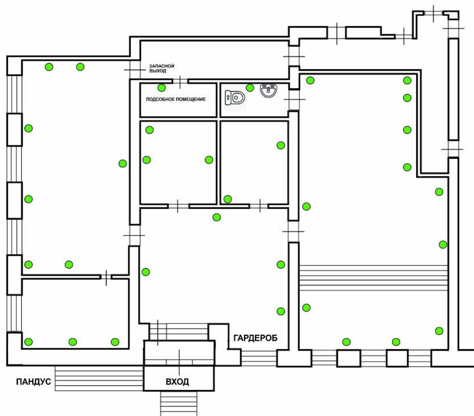
Рисунок 35 – План электрических розеток
