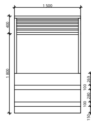
Кубикл вид сбоку
