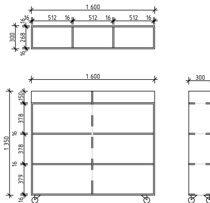
Мобильные стеллажи
