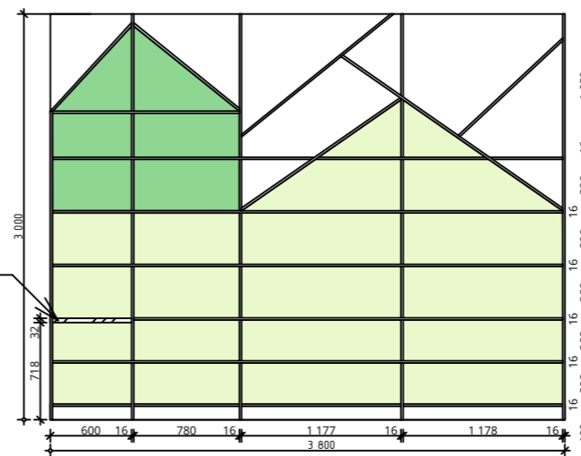
Стеллаж Тип 1
