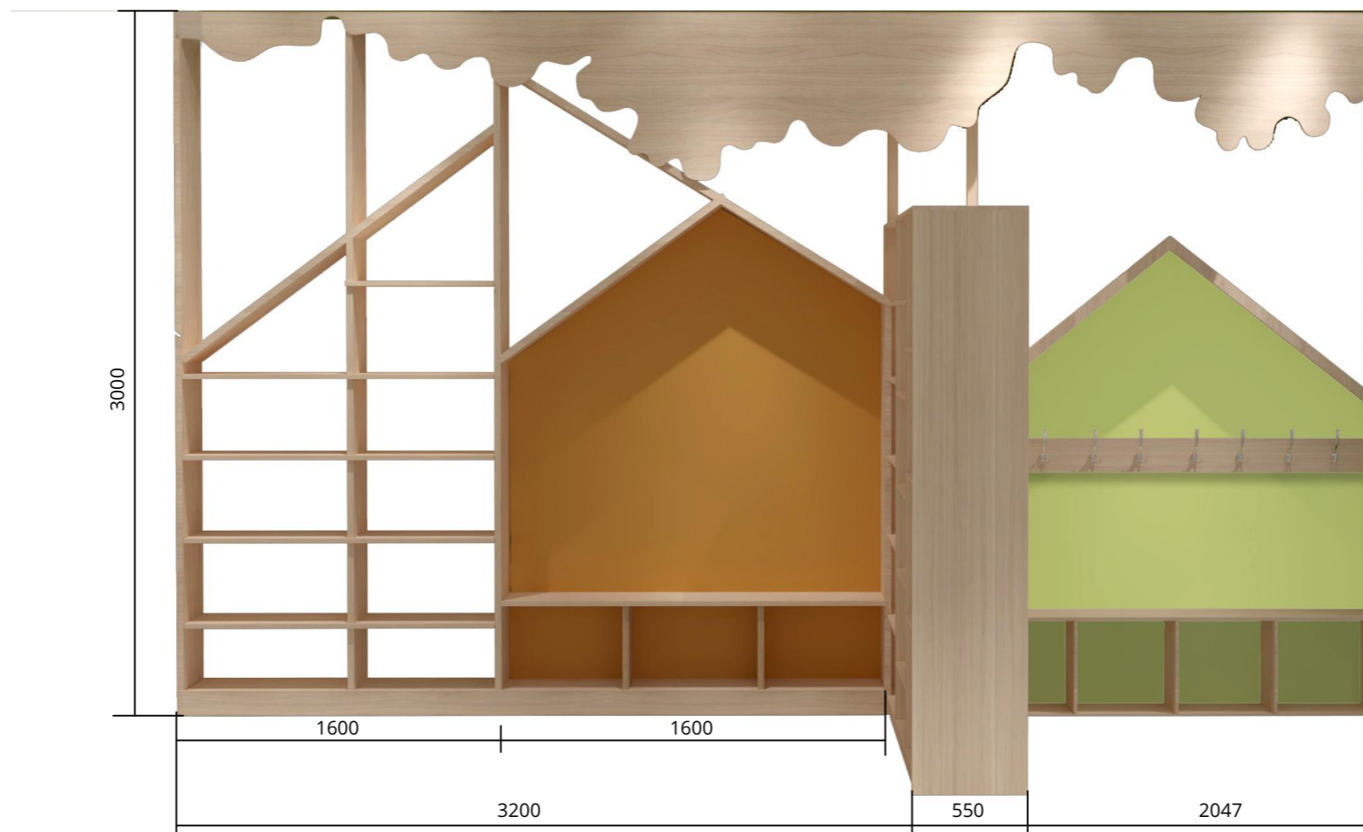
Мобильные стеллажи
