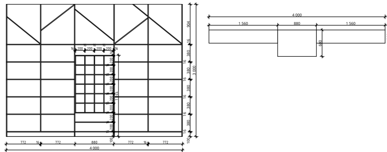
Стеллаж Тип 3
