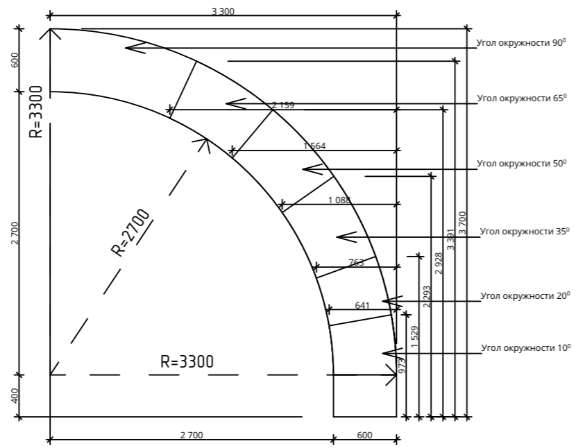
Стеллаж радиусный вид сверху
