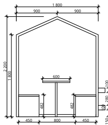
Кубикл вид спереди
