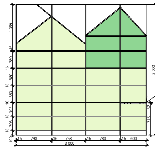
Стеллаж Тип 2
