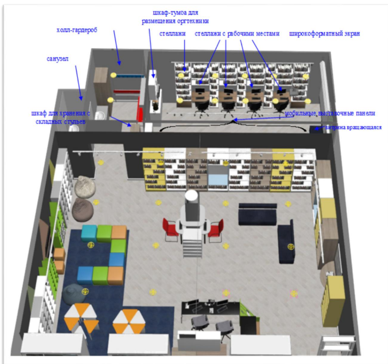
Рис. 3. Зона – трансформер.
