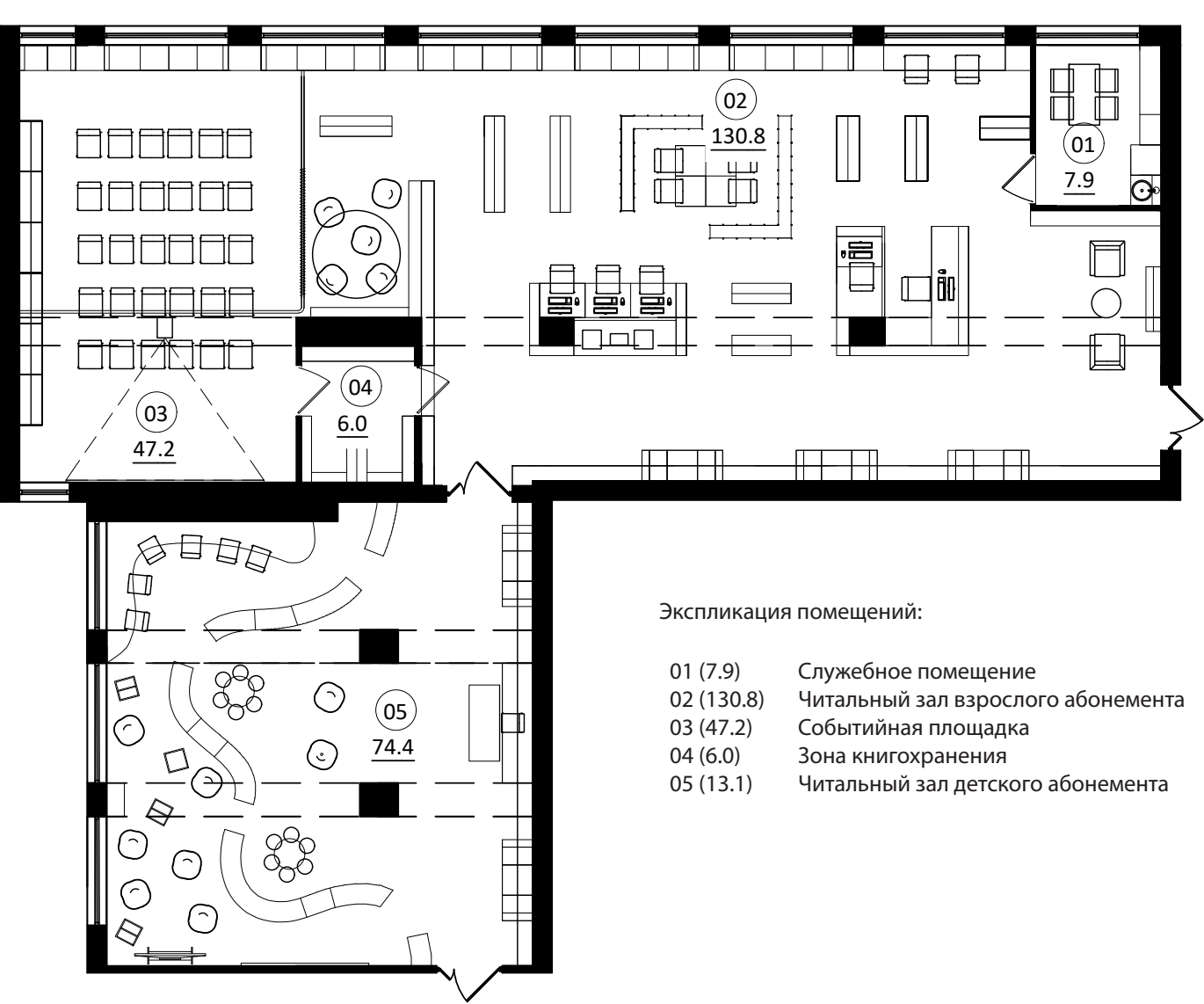
план событийной площадки в режиме проведения презентаций и кинопоказов
