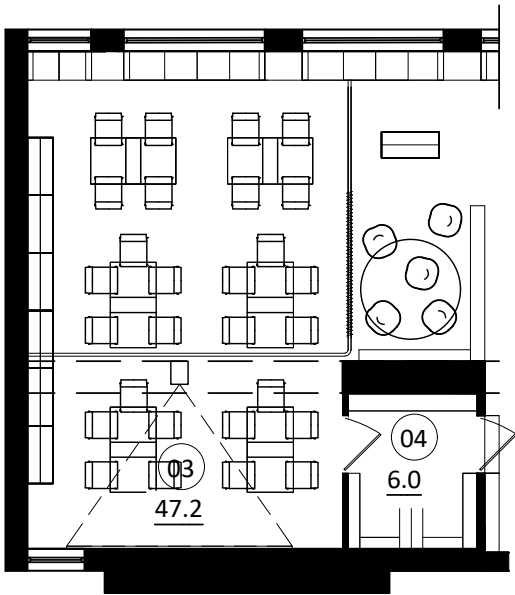
план событийной площадки в режиме проведения мастер-классов и тренингов
