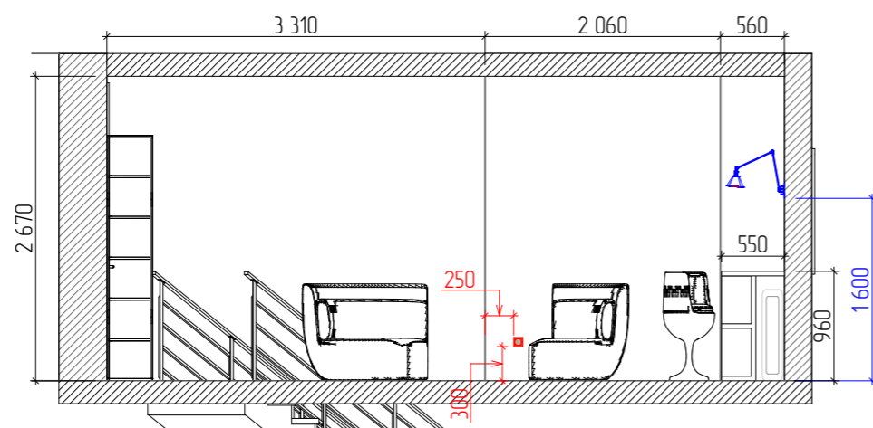
Разрез 9-9
