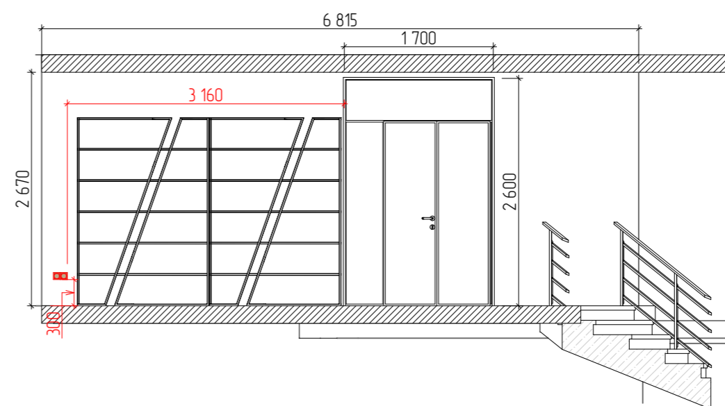
Разрез 12-12
