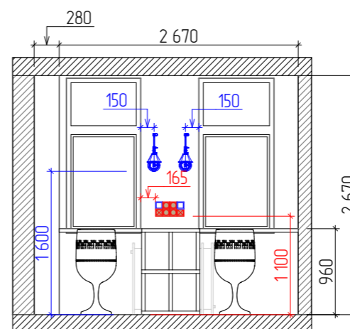
Разрез 10-10
