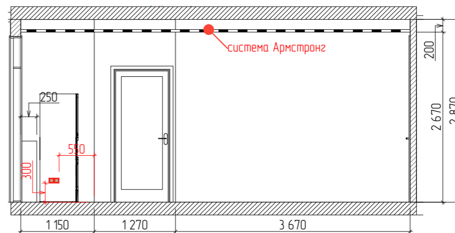
Разрез 2-2
