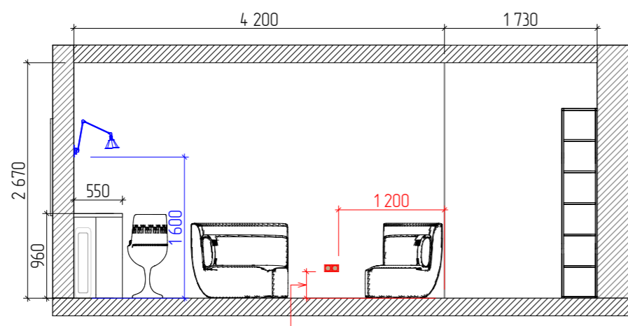
Разрез 11-11
