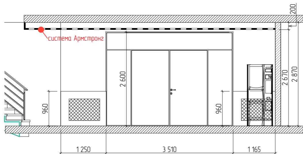
Разрез 1-1
