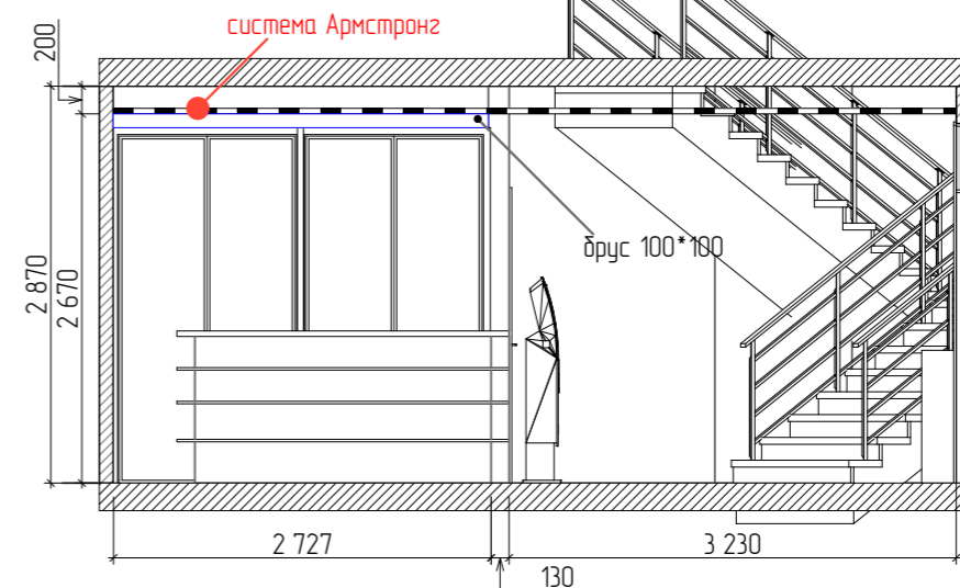
Разрез 4-4
