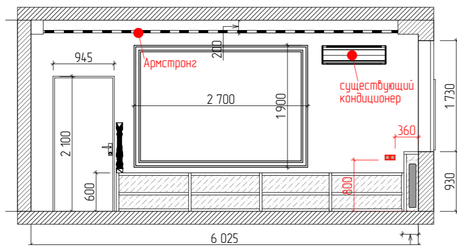
Разрез 16-16
