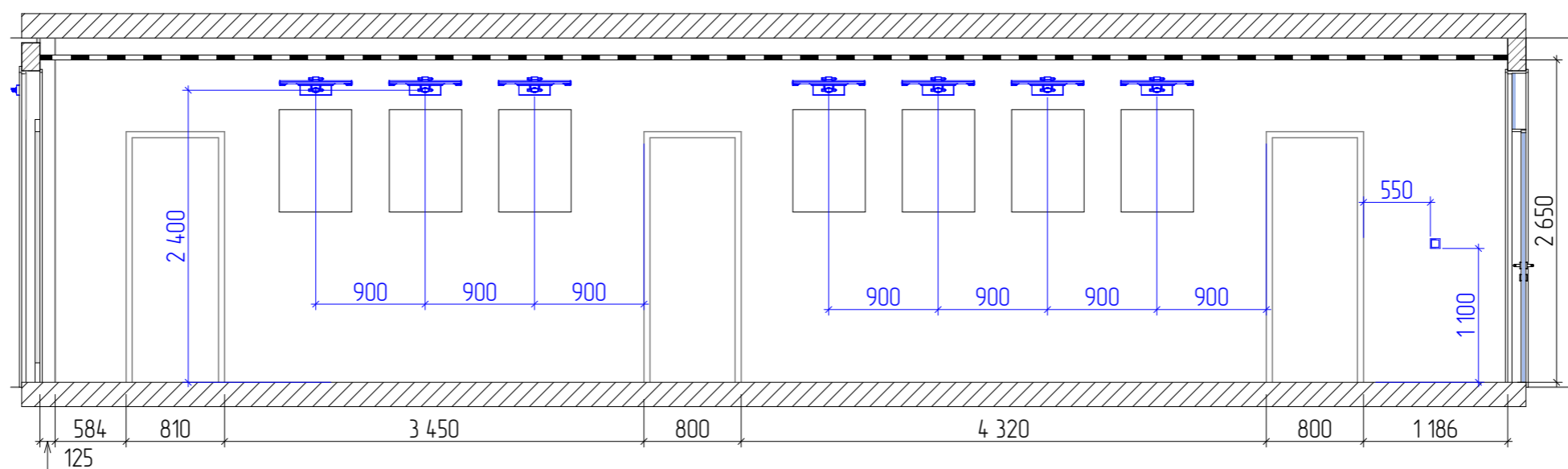
Разрез 14-14
