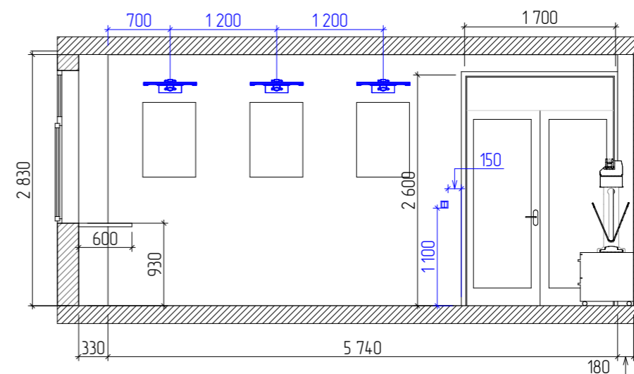
Разрез 22-22
