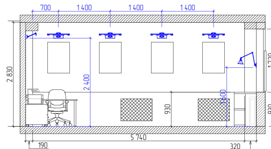
Разрез 20-20
