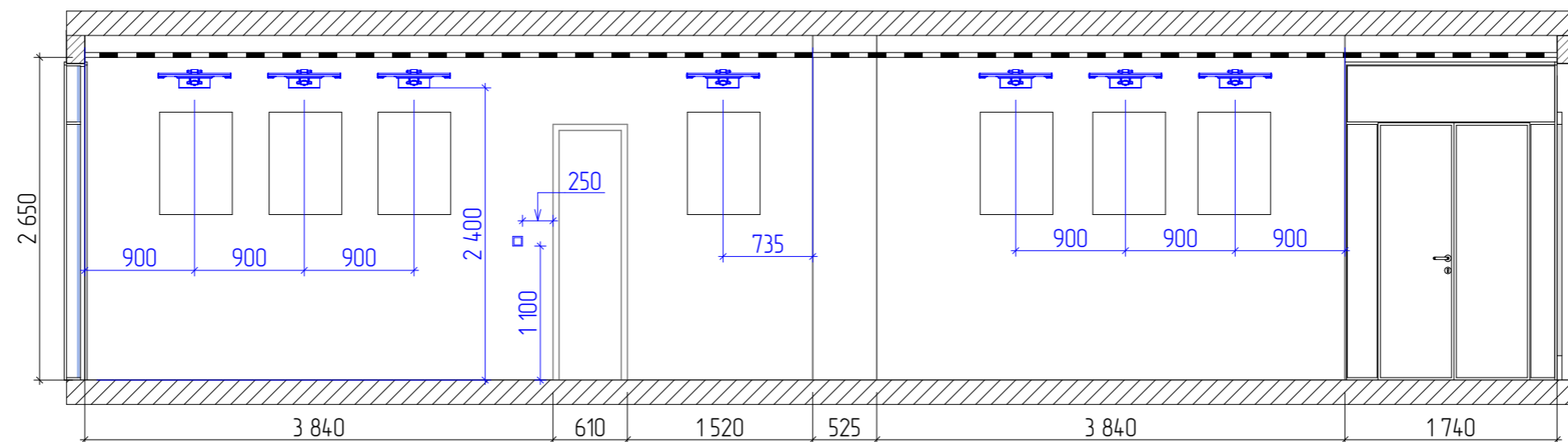
Разрез 13-13
