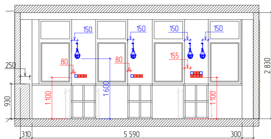
Разрез 21-21
