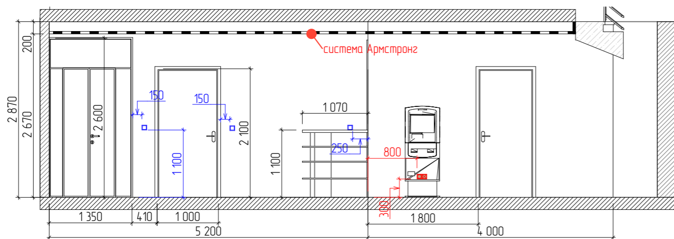
Разрез 3-3
