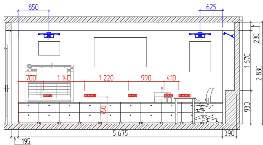
Разрез 19-19
