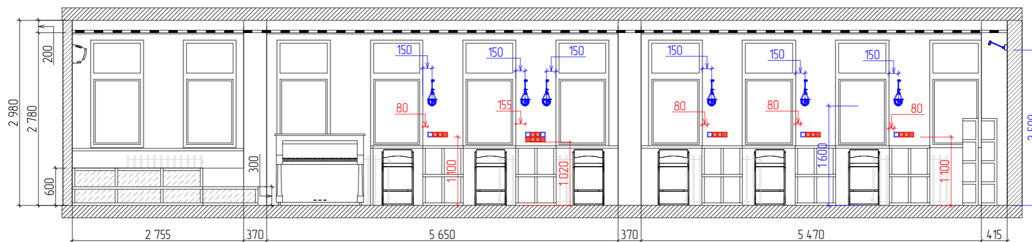
Разрез 18-18
