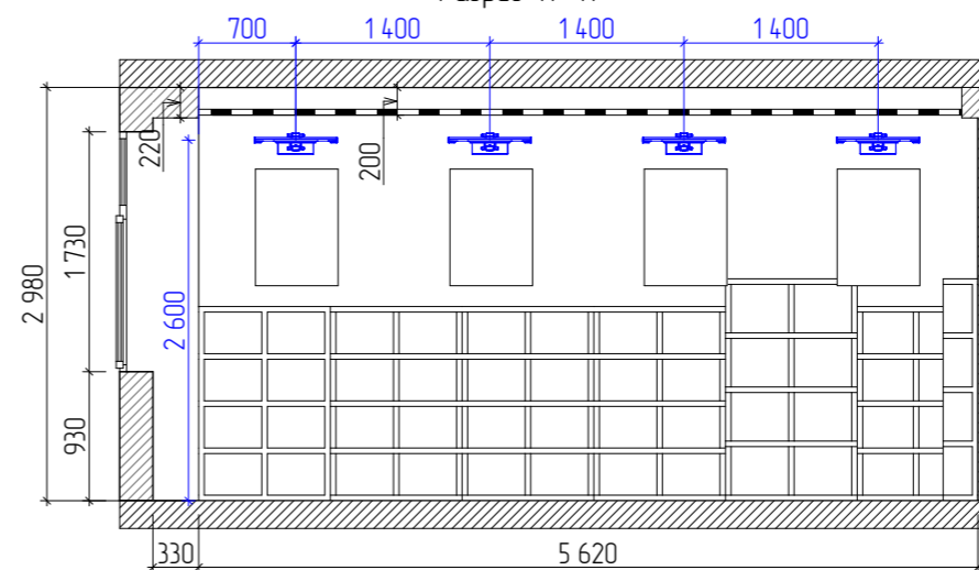
Разрез 17-17
