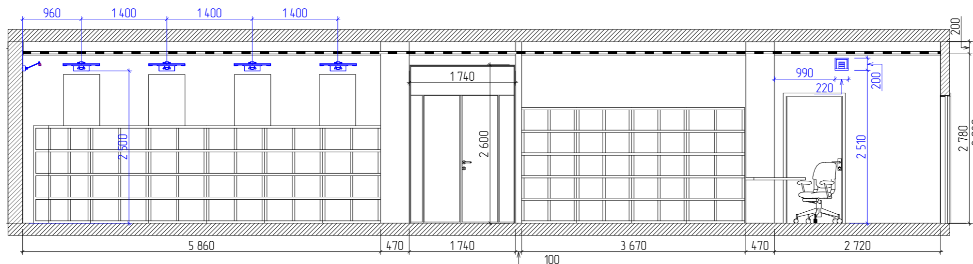
Разрез 18-18
